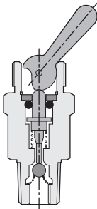
V: Toggle lever type
